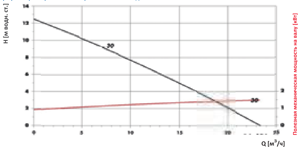
График характеристических кривых насосов модели F 640 PP-30 TR
