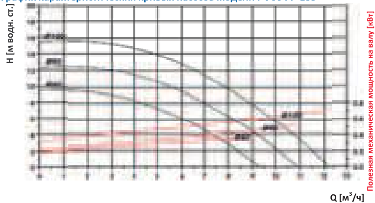
График характеристических кривых насосов модели F 706 PP-185
