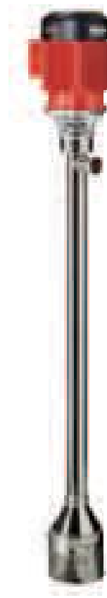
F 620 S-30 с сетчатым фильтром со стороны всаса
