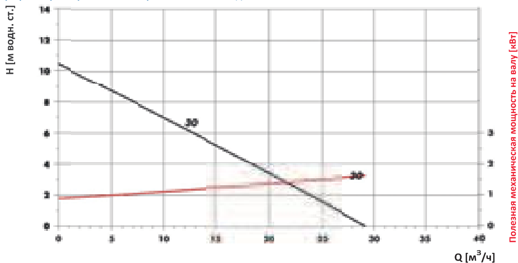
График характеристических кривых насосов модели F 640 PP-230 TR
